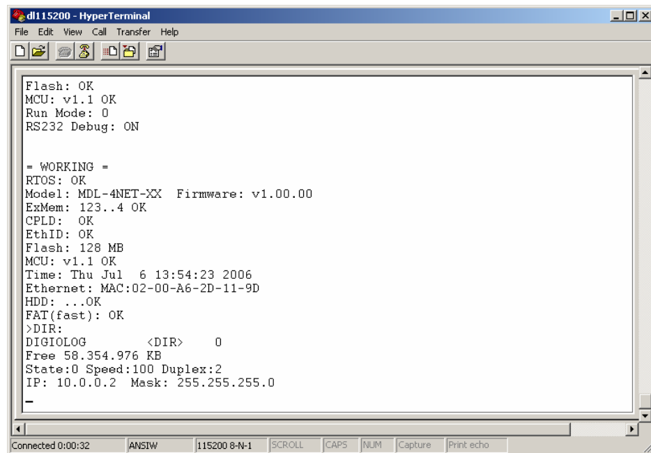
Рисунок 18. Лог через RS-232
