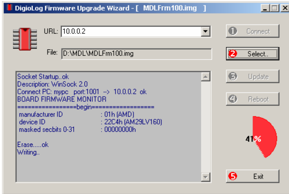
Рисунок 17. Процесс обновления прошивки. ПО «Flasher».
