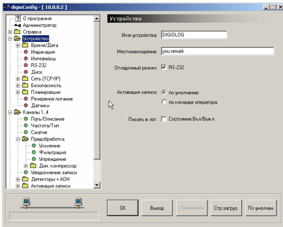
Рисунок 16. Интерфейс программы «DigioConfig».
