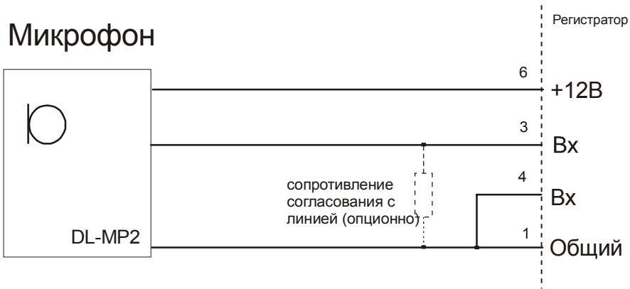
Рисунок 13. Схема подключения микрофона с питанием от регистратора.
