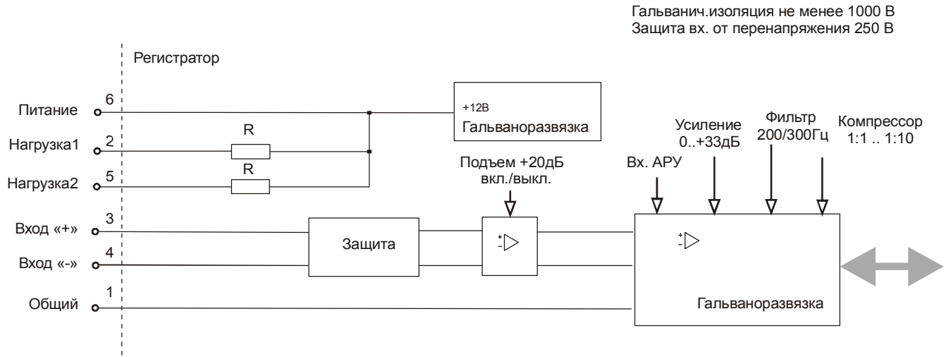
Рисунок 10. Схема аудио входов.
