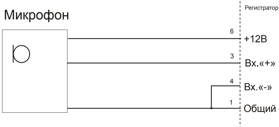
Рисунок 13. Схема подключения микрофона с питанием от регистратора.
