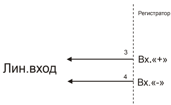
Рисунок 12. Схема подключения к линейному входу.
