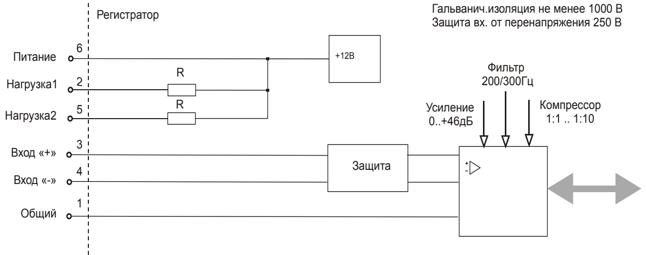
Рисунок 10. Схема аудио входов.
