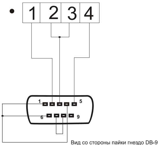
Рисунок 9. Вариант подключения к ПК по RS-232.
