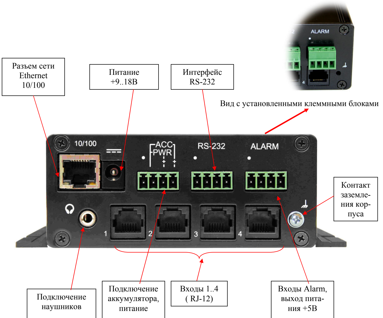
Рисунок 3. Передняя панель устройства (исп. -03).
