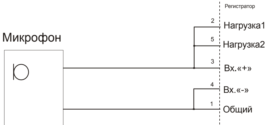
Рисунок 14. Схема подключения микрофона с фантомным питанием +12В.
