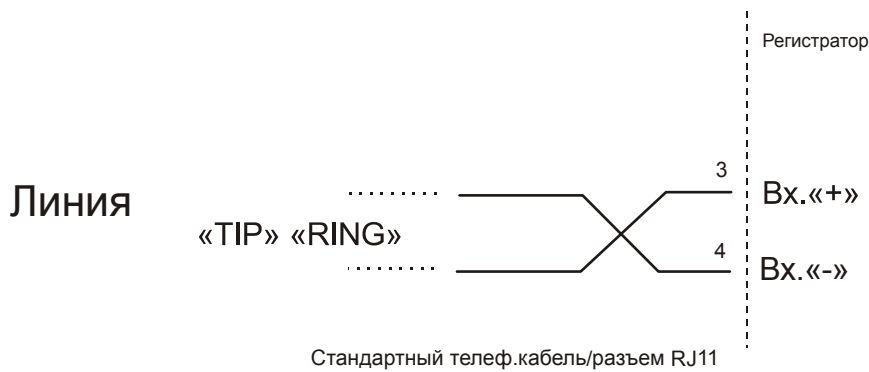
Рисунок 11. Схема подключения к телефонной линии.
