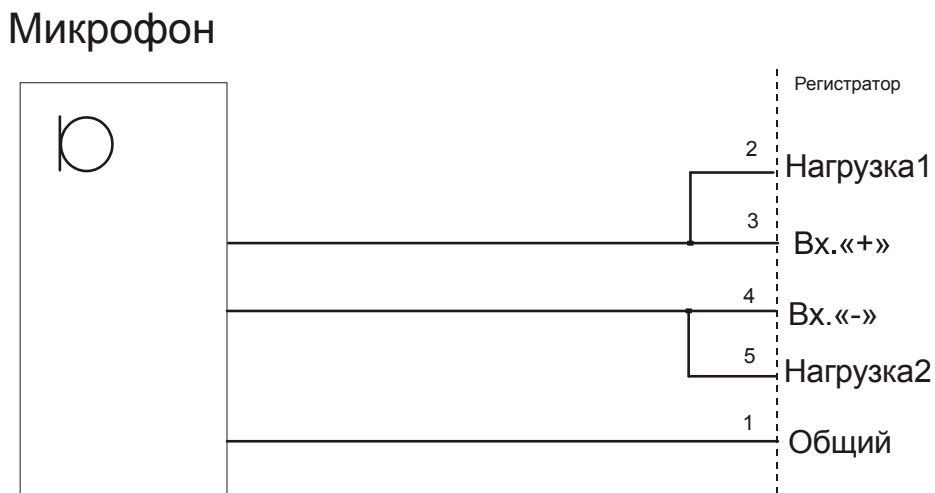
Рисунок 15. Схема подключения балансного микрофона с фантомным питанием +12В.
