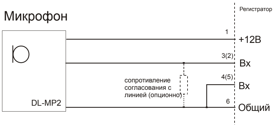
Рисунок 15. Схема подключения микрофона с питанием от регистратора.
