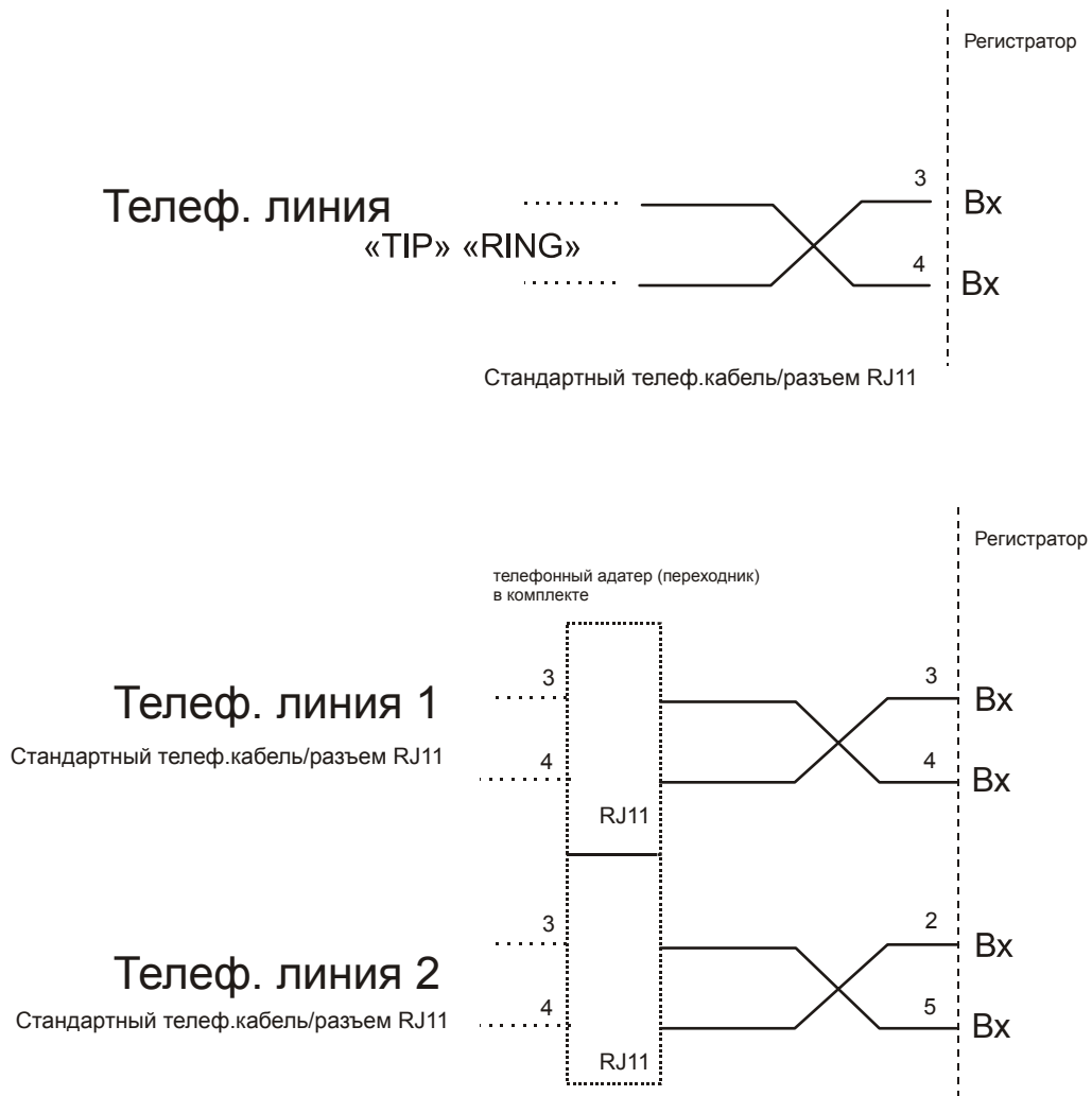
Рисунок 13. Схема подключения к телефонной линии.
