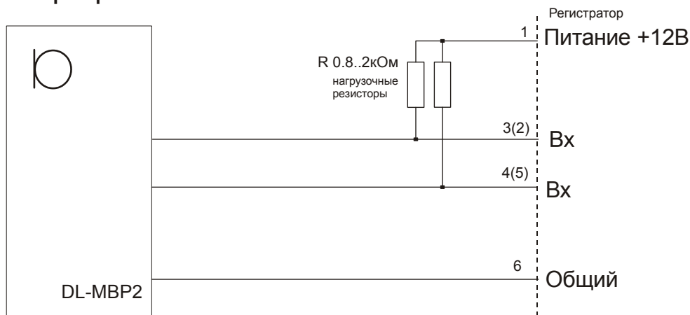
Рисунок 18. Схема подключения балансного микрофона с фантомным питанием +12В.
