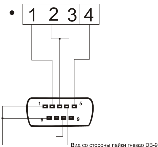
Рисунок 11. Вариант подключения к ПК по RS-232.
