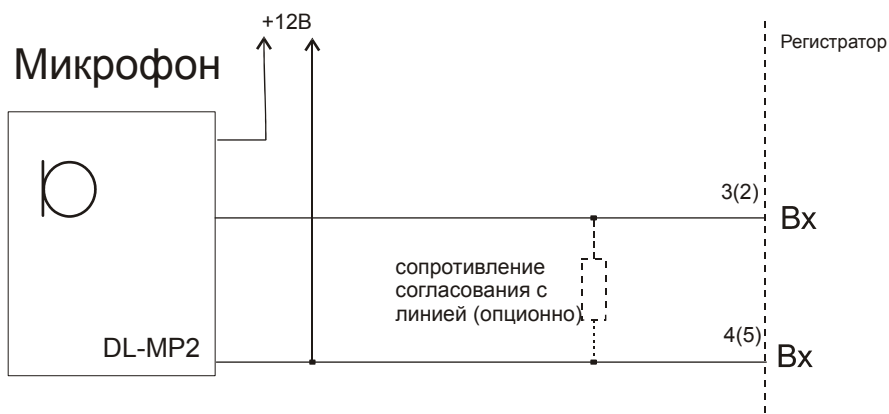
Рисунок 16. Схема подключения микрофона с питанием от внешнего источника.
