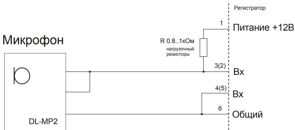
Рисунок 17. Схема подключения микрофона с фантомным питанием +12В.
