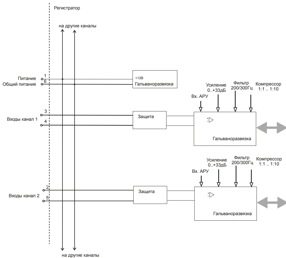
Рисунок 12. Схема аудио входов.
