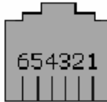
Рисунок 9. Гнездо RJ-12.
