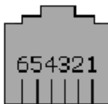
Рисунок 7. Гнездо RJ-12.
