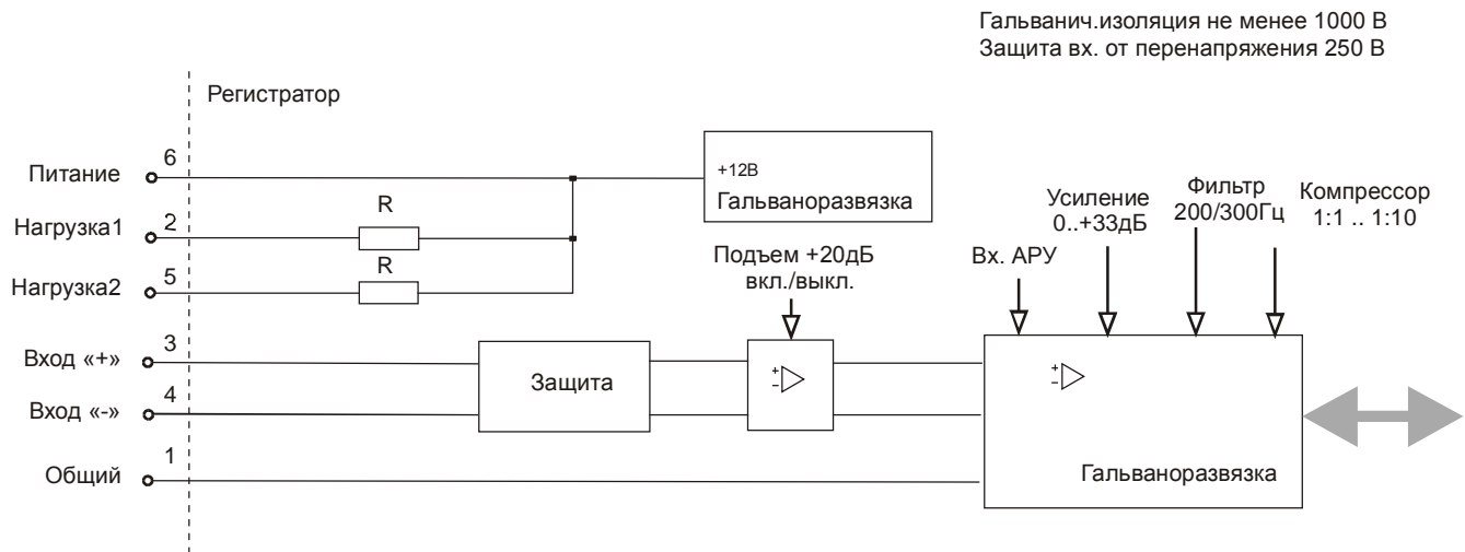
Рисунок 9. Схема аудио входов.
