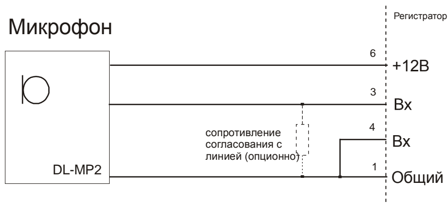
Рисунок 12. Схема подключения микрофона с питанием от регистратора.
