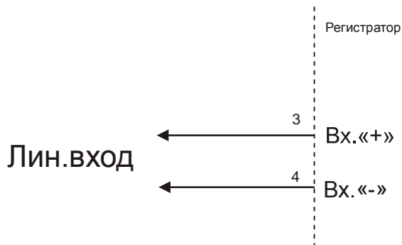
Рисунок 11. Схема подключения к линейному входу.
