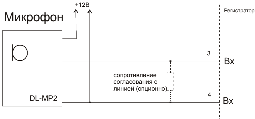
Рисунок 13. Схема подключения микрофона с питанием от внешнего источника.
